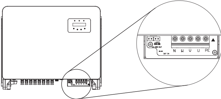
Figura 5.19 fiação
