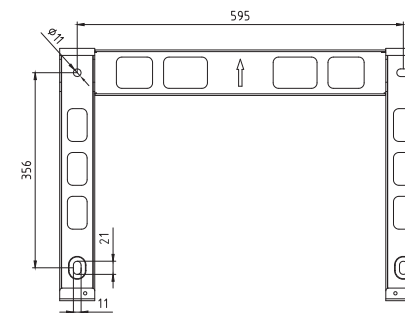
Figura 5.3 Montagem do inversor na parede
