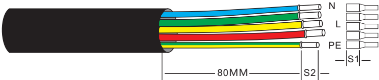
Figura 5.18 Descascar o cabo AC
