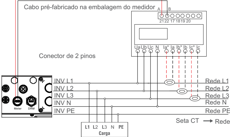
Figura 5.27 Medidor externo do tipo CT - "Medidor na rede"
