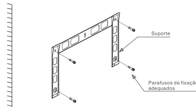
Figura 5.4 Montagem do inversor na parede
