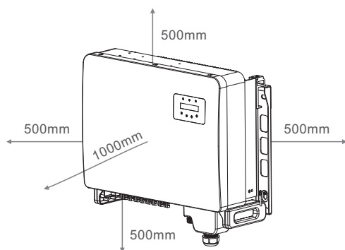
Figura 5.2 Folga de montagem do inversor
