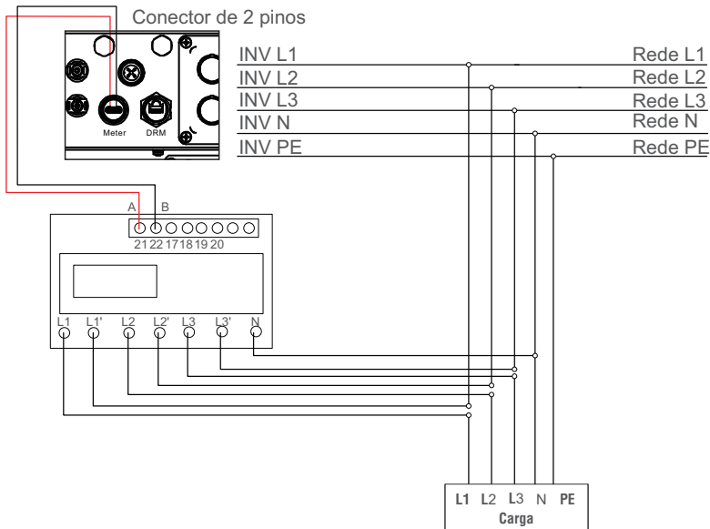
Figura 5.26 Medidor do tipo de inserção direta - "Medidor em carga"
