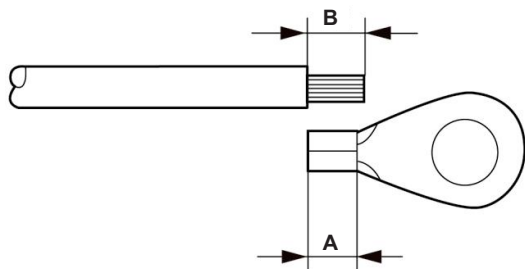
Figura 5.7 Comprimento adequado
