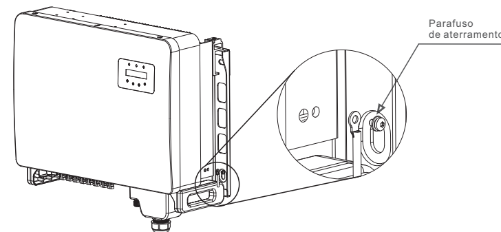
Figura 5.9 Cabo fixo
