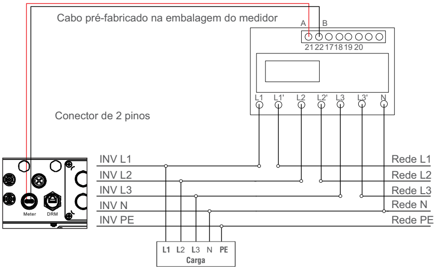
Figura 5.25 Medidor do tipo inserção direta - "Medidor em rede"
