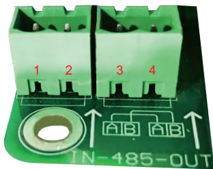
Figura 5.22 Definição do terminal Rs485
