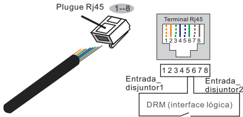
Figura 5.30 Retire a camada de isolamento e conecte-a ao plugue Rj45
