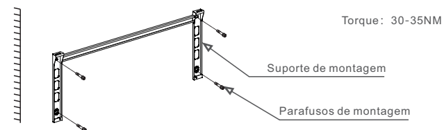
Figura 3.9 Montagem do inversor na parede
