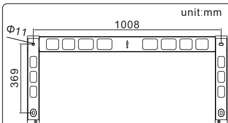
Figura 3.5b Montagem na parede do inversor (ambos com interruptor AC)
