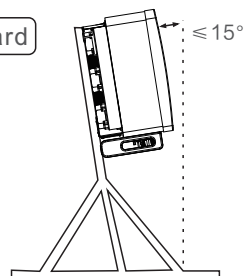
Figura 3.11 Ângulo de instalação correto
