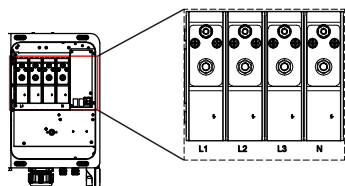
Figura 3.29 Fiação com neutro
