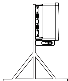
Figura 3.11 Ângulo de instalação correto
