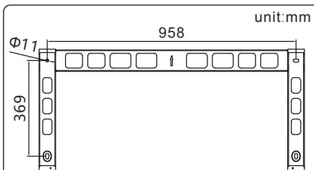
Figura 3.5a Montagem na parede do inversor
