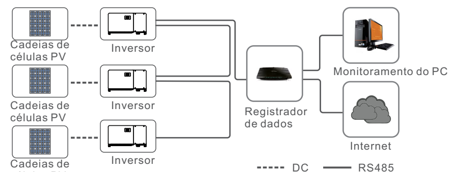
Figura 4.1 Sistema de monitoramento de vários inversores (Rs485)
