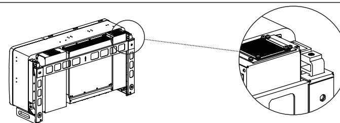
Figura 3.10 Instalação do inversor
