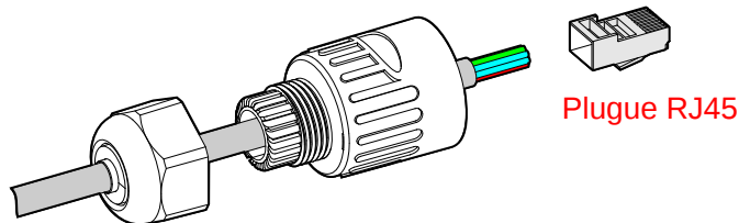
Figura 3-30 Crimpe os cabos do plugue RJ45
