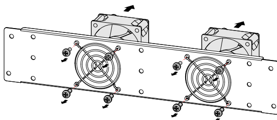
Figura 5-3 Desmonte o ventilador
