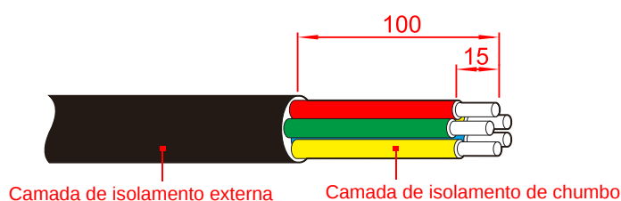
Figura 3-23 Desencape o fio de saída de CA (unidade: mm)
