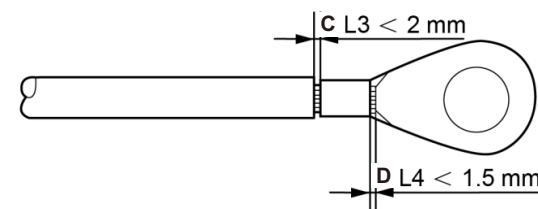
Figura 3.18 Desencapar fio
