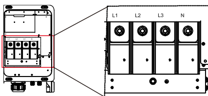
Figura 3.29 Fiação com neutro
