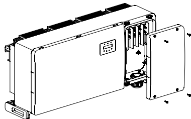
Figura 3.28 Remova a tampa da caixa de junção
