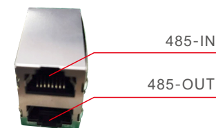
Figura 4.2 Porta RJ45
